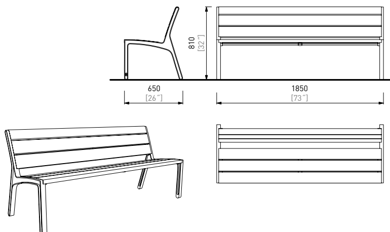
Lavička mmcité MIELA 151_2D
